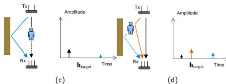
รูปที่ 2.6 แผนภาพช่องสัญญาณเป้าหมาย ในลักษณะสัญญาณตกค้างเชิงผลต่าง กรณีเป้าหมายบดบัง
