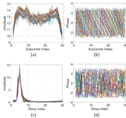
รูปที่ 2.7 กราฟเปรียบเทียบข้อมูล CSI ดิบในโดเมนความถี่ กับโดเมนดีเลย์ทั้งแอมพลิจูดและเฟส
