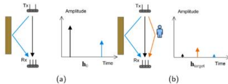
รูปที่ 2.5 แผนภาพช่องสัญญาณพื้นหลัง และช่องสัญญาณเป้าหมายกรณีเป้าหมายก่อให้เกิดพาราสสะท้อนเพิ่มเติม [2]
